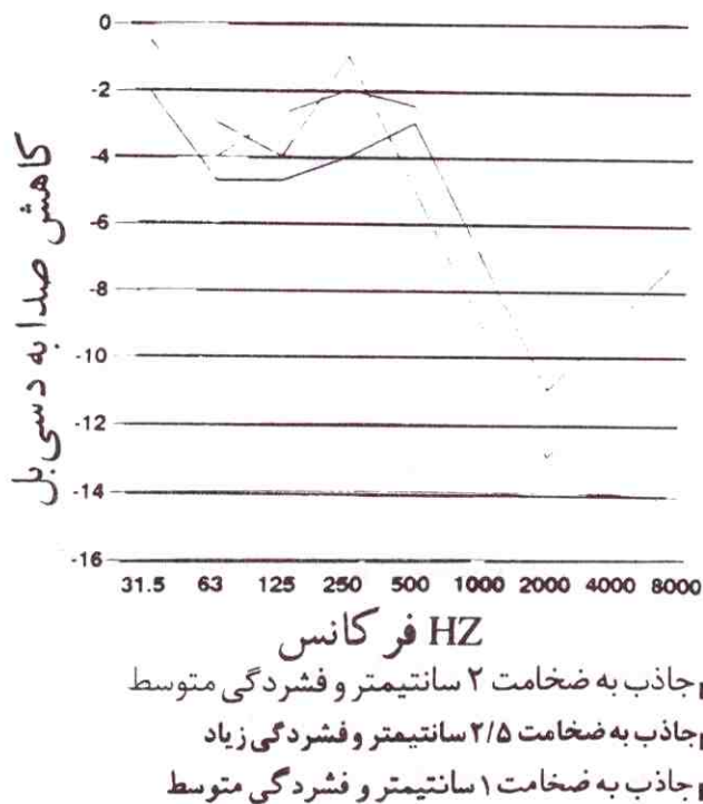
نمودار ۱- کاهش صدای فرکانس های مختلف در درون محفظه سیستم لیندلی با جاذب های مختلف
