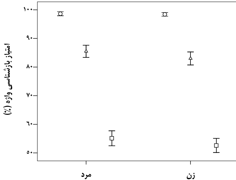
نمودار ۱- میانگین و انحراف معیار امتیاز آزمون گفتار با فشردگی زمانی در ۳ نسبت مورد بررسی در دو جنس. (O: نسبت فشردگی ۰٪، +: نسبت فشردگی ۴۰٪، Δ: نسبت فشردگی ۶۰٪، □: نسبت فشردگی ۷۰٪).
