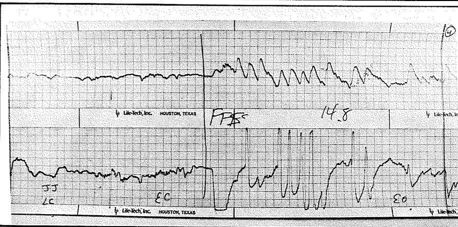
تصویر ۲: آزمایش کالریک با آب سرد در گوش چپ (۳۰°) به نیستاکموس با شدت و دامنه زیاد در حالت چشمان باز توجه کنید.
