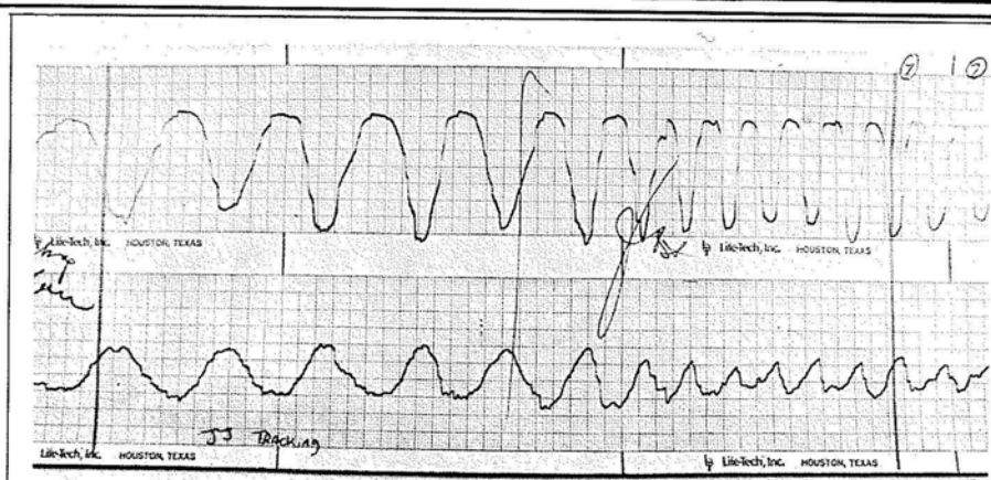
تصویر ۴: ردیابی سینوسی، یک الگوی یکنواخت (Smooth Pattern) کامل را نشان نمی‌دهد و شاید بیشتر شبیه به «Saccadic Pursuit» باشد، اما اساساً در محدوده طبیعی است. (Bitemporal Leads - الکترودهای افقی)
