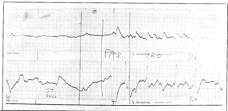
تصویر ۳: آزمایش کالریک با آب گرم در گوش راست (۴۲°) مجدداً عدم توانایی در سرکوب نیستاکموس توسط تثبیت بصری بارز را بیان می کند. (Bütemporal Leads - الکترودهای افقی)
