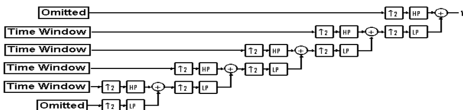
شکل ۸- بانک فیلتری برای سنتز سیگنال گسیل‌های صوتی برانگیخته گذرا بعد از اعمال پنجره‌های زمانی
