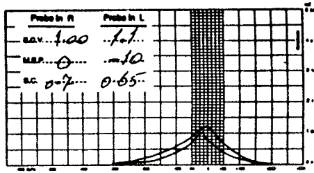
شکل ۳- ایمیتانس ادیومتری
