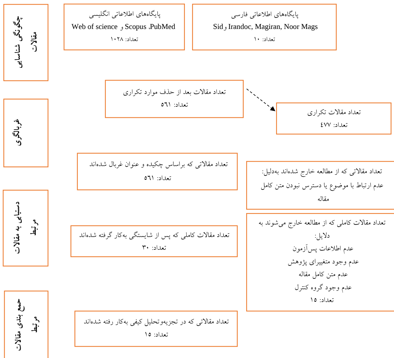
شکل ۱- فلوجارت جست‌وجو
