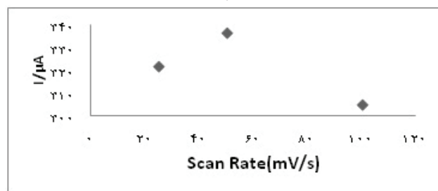
شکل ۶- ولتاموگرام‌های تمایز پالسی پاسخ الکتروکود تغییر یافته برای بهینه سازی زمان (الف) (۱۰، ۲۰، ۳۰، ۴۰، ۵۰، ۶۰، ۷۰، ۸۰، ۹۰) (الف) (ب) پتانسیل (۱/۲۲/۲، ۱/۲۵/۱، ۱/۲۷، ۱/۳۰، ۱/۳۵، ۱/۴۰ ولت)، (ج) سرعت خوانش (۵۰، ۲۵ و ۱۰۰ mV/s) (ثانیه)
