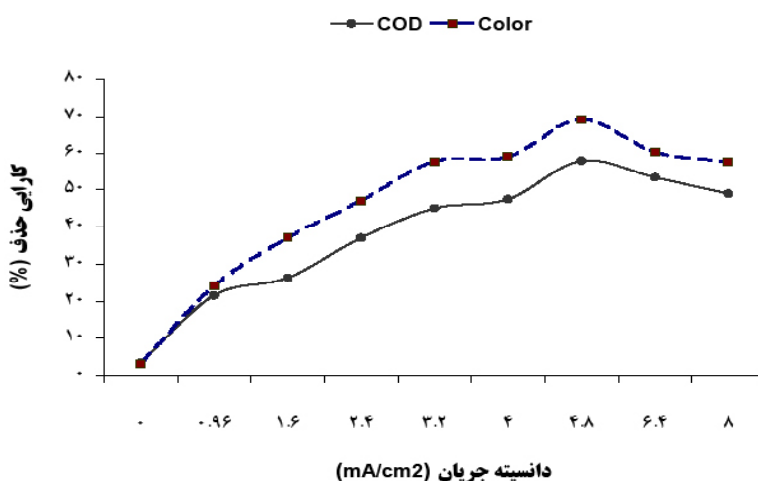
شکل ۴: اثر دانسیته جریان بر کارایی حذف COD و رنگ به وسیله فرایند الکتروفتون در فاضلاب واقعی نساجی بر پایه رنگ اسیدی (هوای ورودی غلظت یون فرو ۱/۵ L/min، pH=۳، ۲ m mol و زمان واکنش ۱۶۰ min)
