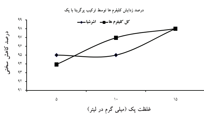
شکل ۶: راندمان زدایش کلیروم ها
