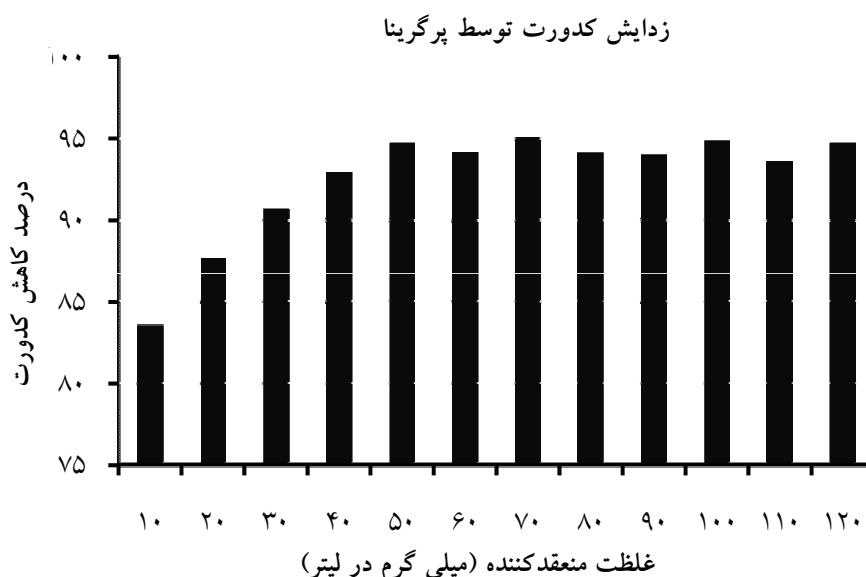
شکل ۱: درصد کاهش کدورت در غلظت‌های متفاوت پرگرینا
