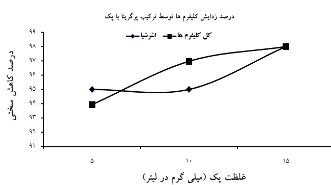
شکل ۶: راندمان زدایش کلیروم ها
