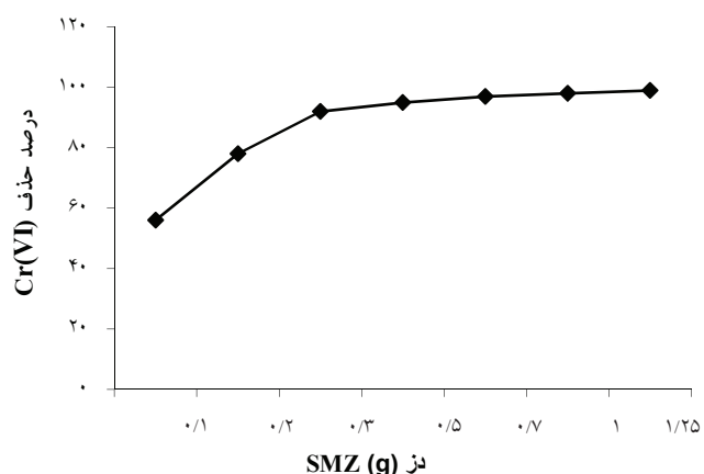
شکل ۲: تاثیر تغییرات دز جاذب SMZ بر کارایی حذف Cr(VI) در C Cr = ۱ mg/L و pH=۷
