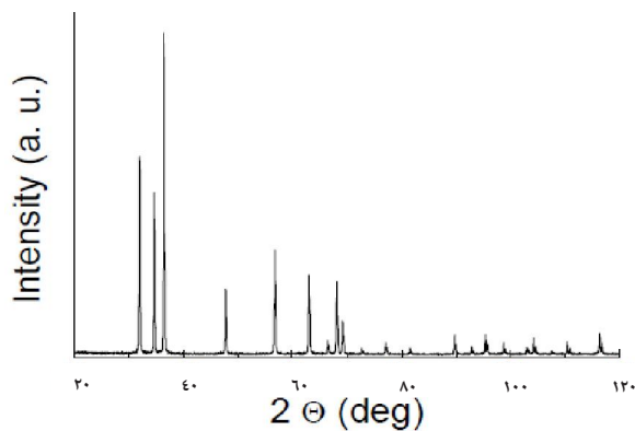
XRD !
