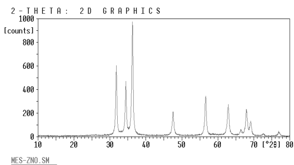
شکل ۲: نمودار XRD نانو اکسید روی
