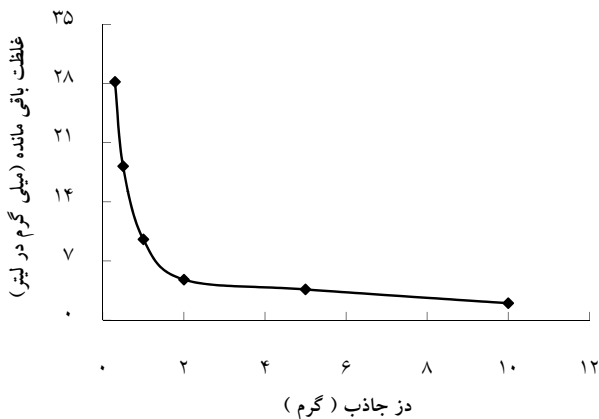
شکل ۶: تاثیر دز جاذب در جذب رنگ متیلن بلوغلظت ثابت 200 میلی گرم در لیتر (pH اولیه ۹)
