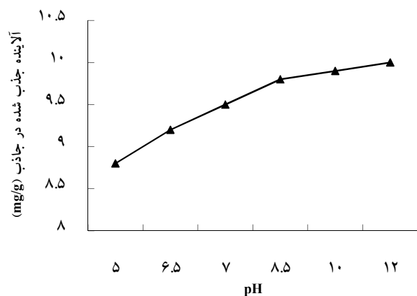
شکل ۵: تاثیر pH اولیه در جذب رنگ با غلظت ثابت 200 میلی گرم در لیتر (دز جاذب 1 \text{ گرم} )
