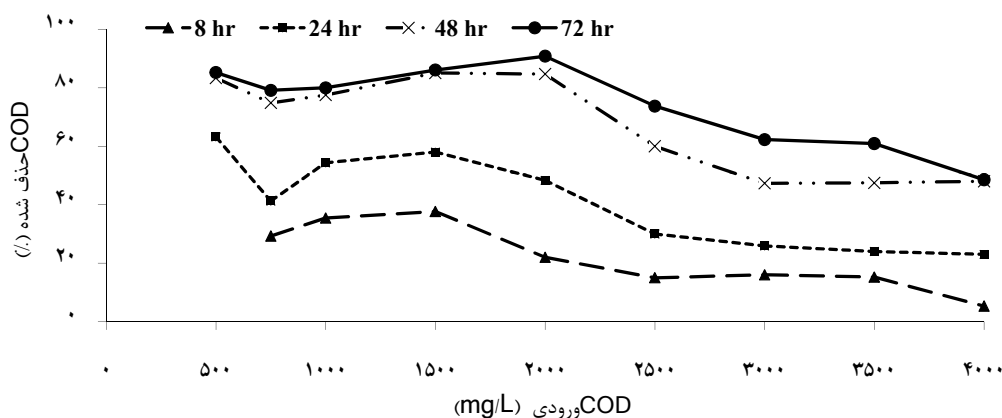
شکل ۳: راندمان حذف آنیلین در زمان‌های ماند مختلف با پرشدگی ۵۰ درصد
