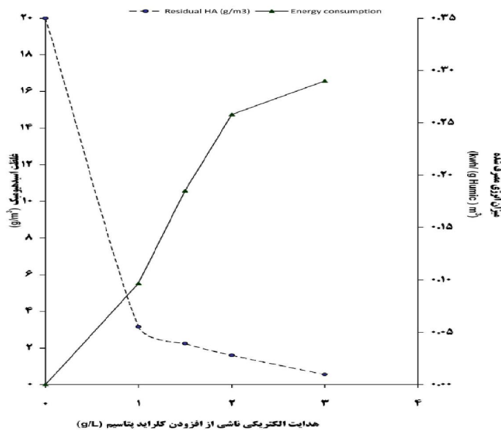
شکل ۶: اثر هدایت‌های الکتریکی مختلف بر میزان مصرف انرژی الکتریکی در کاهش غلظت ماده اسید هیومیک (زمان واکنش ۶۰ دقیقه، اختلاف پتانسیل ۱۰ ولت، pH=5 ، اسید هیومیک ۲۰ میلی گرم بر لیتر)
