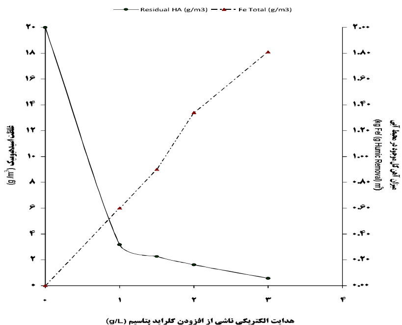
شکل ۷: اثر هدایت‌های الکتریکی مختلف بر مقدار تولید آهن (الکتروود آهن مصرفی) (اختلاف پتانسیل ۱۰ ولت، زمان واکنش ۶۰ دقیقه، pH=5 ، اسید هیومیک ۲۰ میلی گرم بر لیتر)
