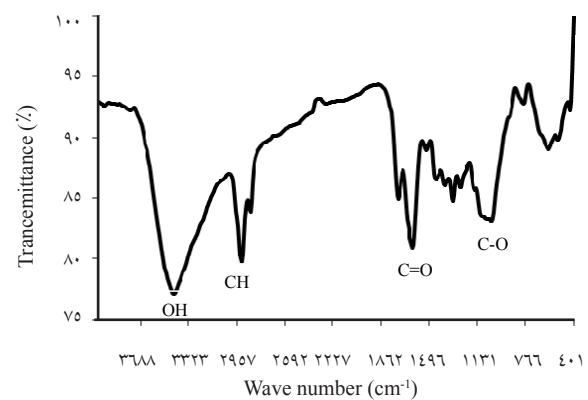
شکل ۲- الف: طول موج FTIR پوست سبز گردو از ۴۰۰ تا cm^{-1}
