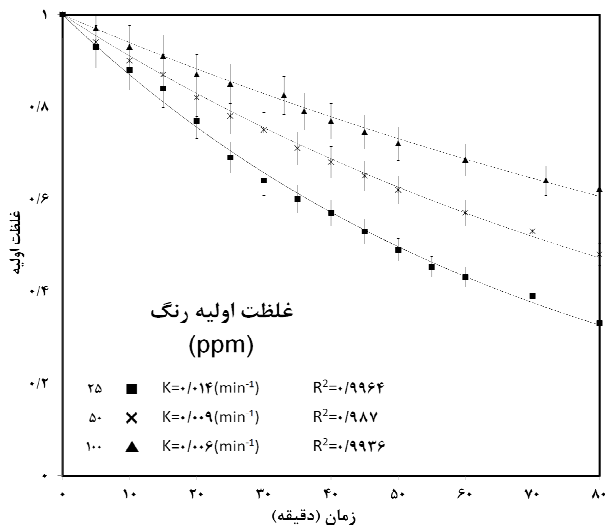
(ب) رنگ‌زدایی رنگ اسیدی سیاه ۲۶ توسط \text{TiO}_2 تثبیت شده برای مقادیر مختلف رنگ‌زا (غلظت رنگ ۵۰ ppm، pH نرمال و غلظت آنیون: ۰ mM)
