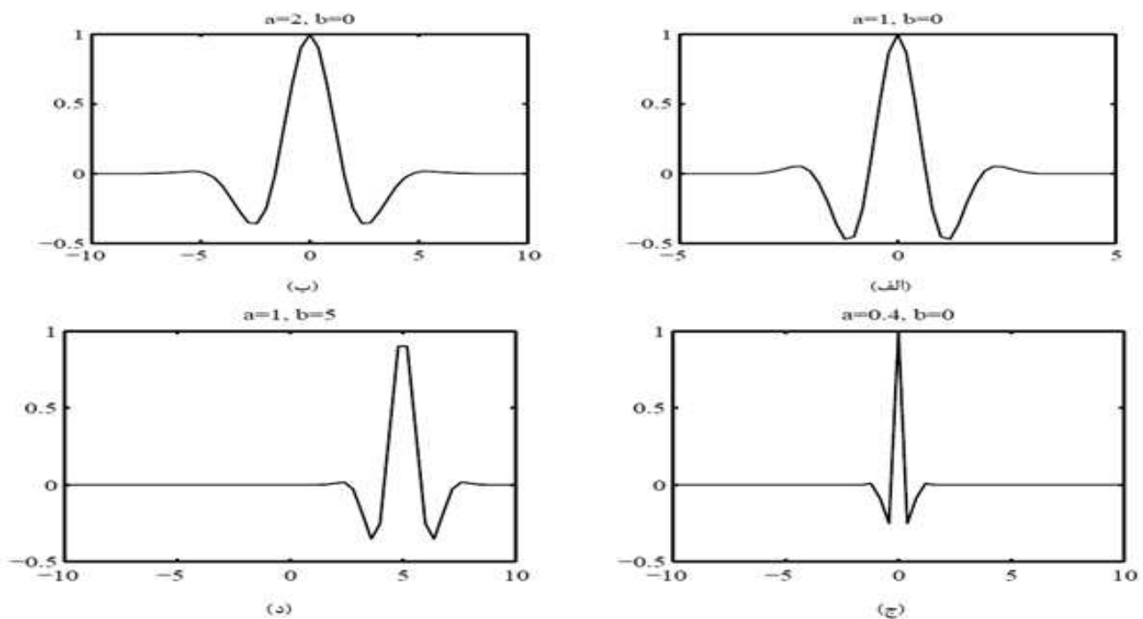
شکل ۲: موجک مورلت
