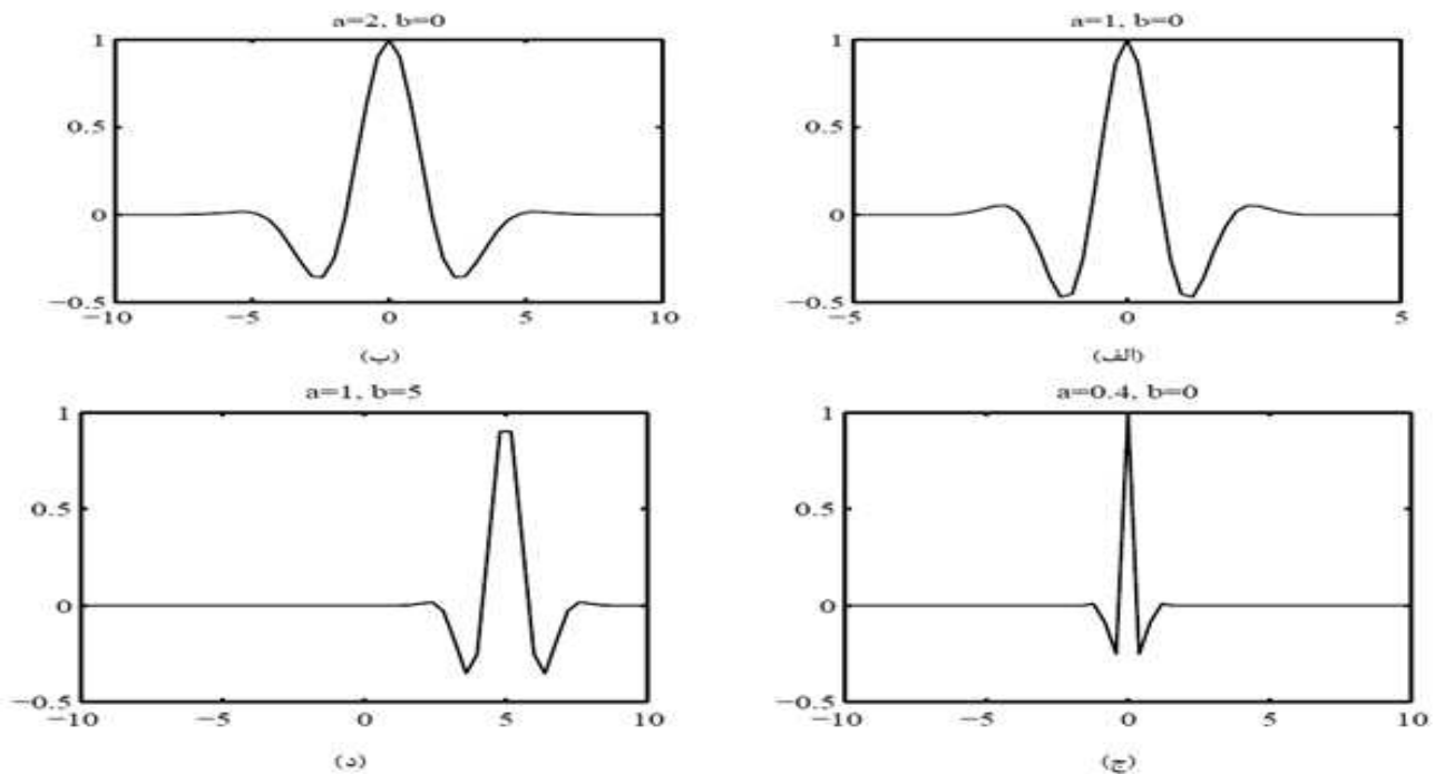
شکل ۲: موجک مورلت
