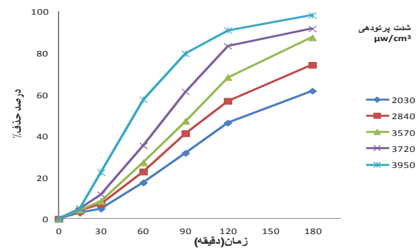
نمودار ۵- تاثیر شدت تابش در حذف اسید هیومیک در فرایند UV/ZnO (در غلظت اولیه 2\text{mg/L} ، pH خنثی)
