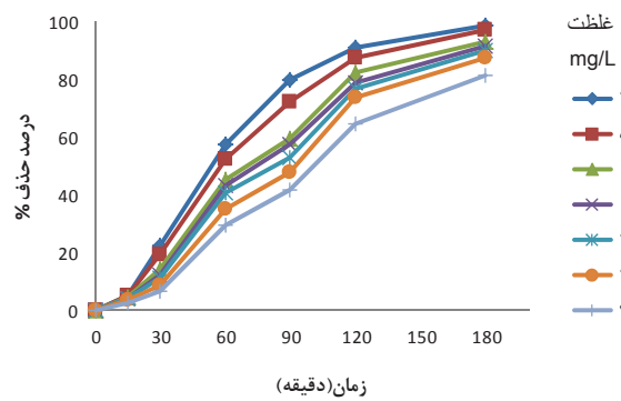
نمودار ۴- تاثیر غلظت اولیه اسید هیومیک و مدت زمان پرتودهی در حذف HA در pH خنثی، شدت پرتودهی 3950\ \mu\text{w/cm}^2
