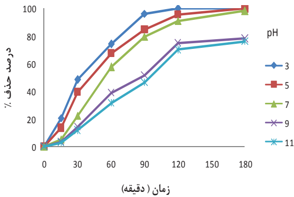
نمودار ۳- تاثیر غلظت اولیه اسید هیومیک و مدت زمان پرتودهی در حذف HA در pH خنثی، شدت پرتودهی 2\text{mg/L} و شدت پرتودهی 3950\ \mu\text{w/cm}^2
