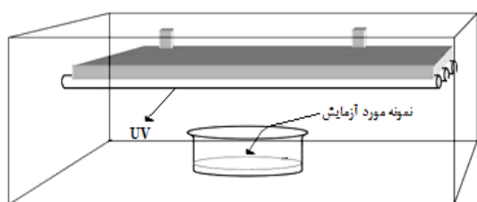
شکل ۲- شماتیک راکتور شیمیایی مورد استفاده
