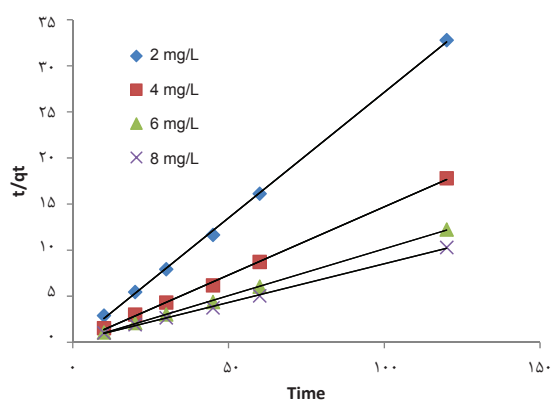
نمودار ۷- مدل سینتیک شبه درجه دو برای جذب فلوراید با استفاده از نانوالومینا پوشش داده شده بر روی نانوتیوب کربنی چندجداره
