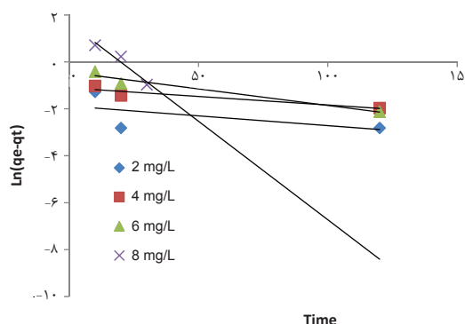
نمودار ۸- مدل سینتیک شبه درجه یک برای جذب فلوراید با استفاده از نانوالومینا پوشش داده شده بر روی نانوتیوب کربنی چند جداره
