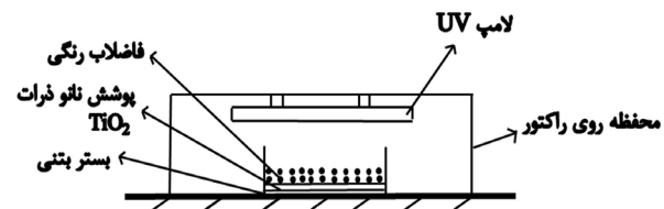
شکل ۲: راکتور مورد استفاده در تحقیق
