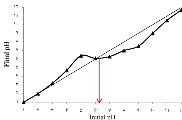
نمودار (۱) تعیین نقطه \text{pH} نقطه صفر (\text{pH}_{\text{ZPC}}) برای نانولوله‌های کربنی
