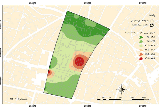
شکل ۳- توزیع فضایی شاخص L_{eq} در روز دوشنبه ۱۳۹۰/۱۲/۱۵
