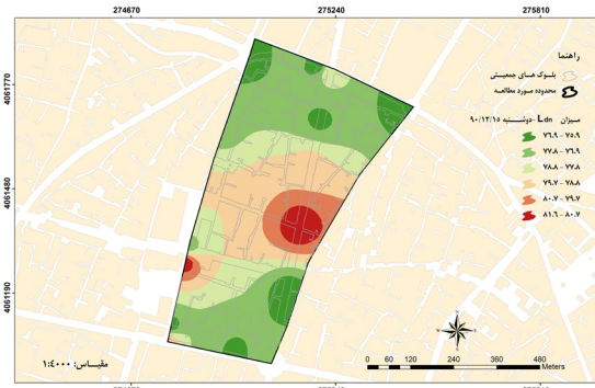
شکل ۴- توزیع فضایی شاخص L_{dn} در روز دوشنبه ۱۳۹۰/۱۲/۱۵
