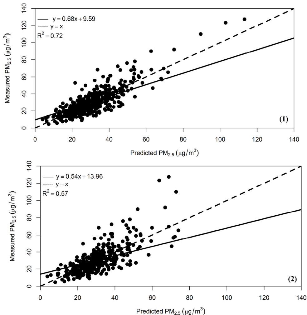
نمودار ۲- مقایسه مقادیر غلظت پیش‌بینی شده و اندازه‌گیری شده (۱) مدل‌سازی (۲) اعتبار‌سنجی
