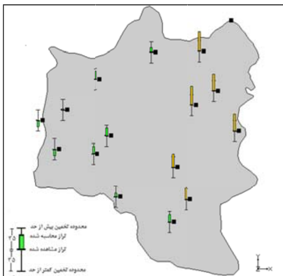
شکل ۵- مقایسه بین سطح آب مشاهده شده و شبیه‌سازی شده
