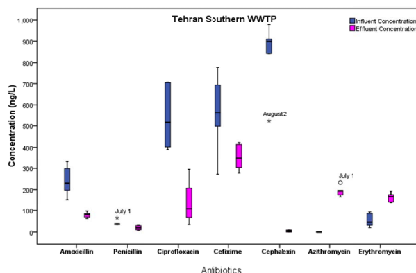
نمودار ۲- Box plot غلظت‌های اندازه‌گیری شده آنتی بیوتیک‌های هدف، در تصفیه خانه فاضلاب جنوب برای نمونه‌های ورودی و خروجی فاضلاب براساس (ماکزیمم، چارک سوم، میانه، چارک اول و مینییم)
