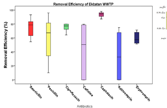
نمودار ۳- کارایی حذف (درصد) آنتی بیوتیک‌های هدف در تصفیه خانه فاضلاب اکباتان براساس (ماکزیمم، چارک سوم، میانه، چارک اول و مینیمم)
