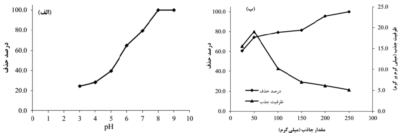
نمودار ۱- (الف) اثر pH بر میزان جذب نیکل (II) توسط جاذب Fe_2O_3 (غلظت اولیه: 50 mg/L ، مقدار جاذب: 0.1 g ، زمان تماس: 30 min ، pH=3-9 ) (ب) اثر مقدار جاذب بر میزان جذب نیکل (II) توسط جاذب Fe_2O_3
