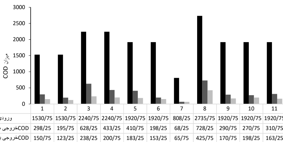
نمودار ۴- COD ورودی و خروجی رنگ راکتیو قرمز ۱۹۸ در سلول متعارف و بافل دار
