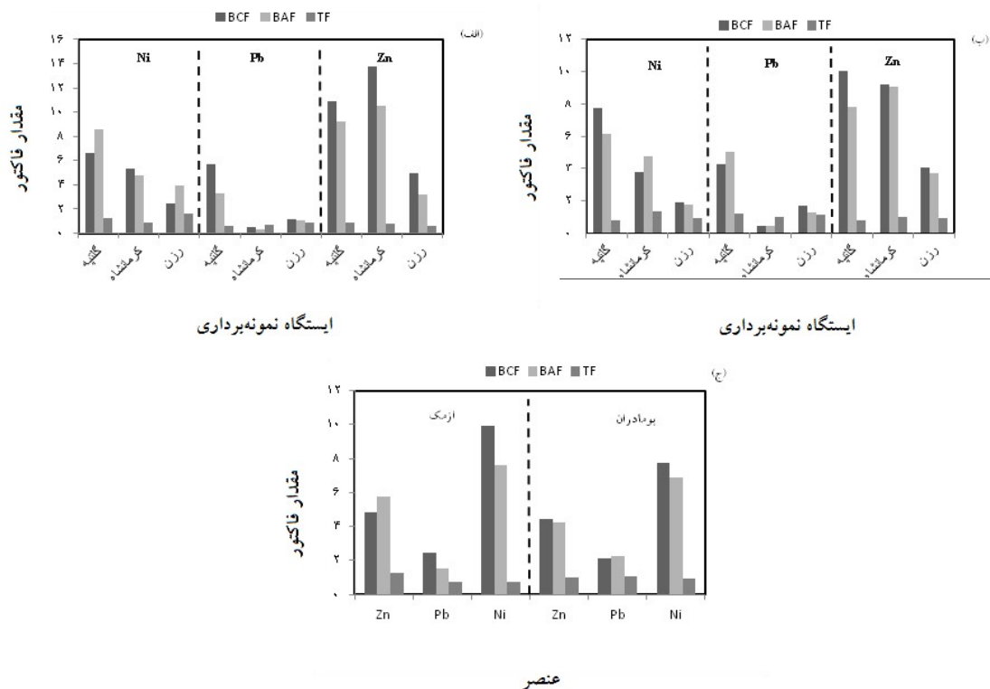
نمودار ۱- (الف) و (ب) به ترتیب مقادیر BCF, BAF, TF عناصر روی، سرب و نیکل در نمونه بافت‌های گیاهی بومادران و ازمک به تفکیک ایستگاه نمونه‌برداری و (ج) میانگین مقادیر BCF, BAF, TF عناصر روی، سرب و نیکل در نمونه بافت‌های گیاهی بومادران و ازمک
