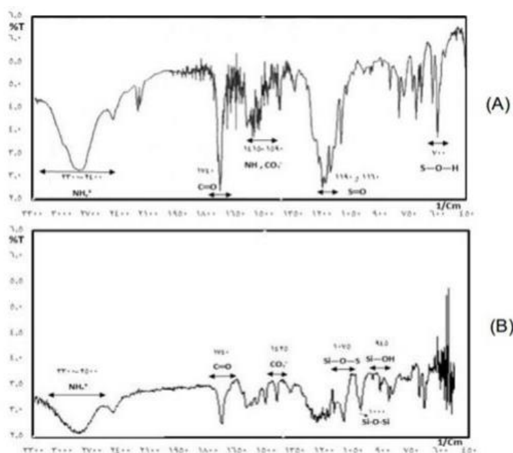
شکل ۲- طیف FTIR مربوط به لیگاند ۵-سولفوآنترانیلیک اسید (A) و FTIR جاذب به همراه تفسیر (B)، تصویر مربوط به FESEM (C) و طیف XRD (D) و آنالیز BET مربوط به جاذب (E)، (F)
