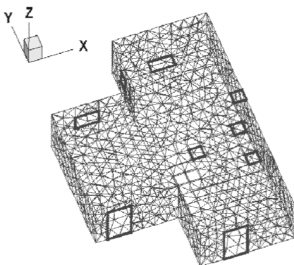
شکل ۲: شبکه بندی ساختمان مسکونی در مدل Fluent
