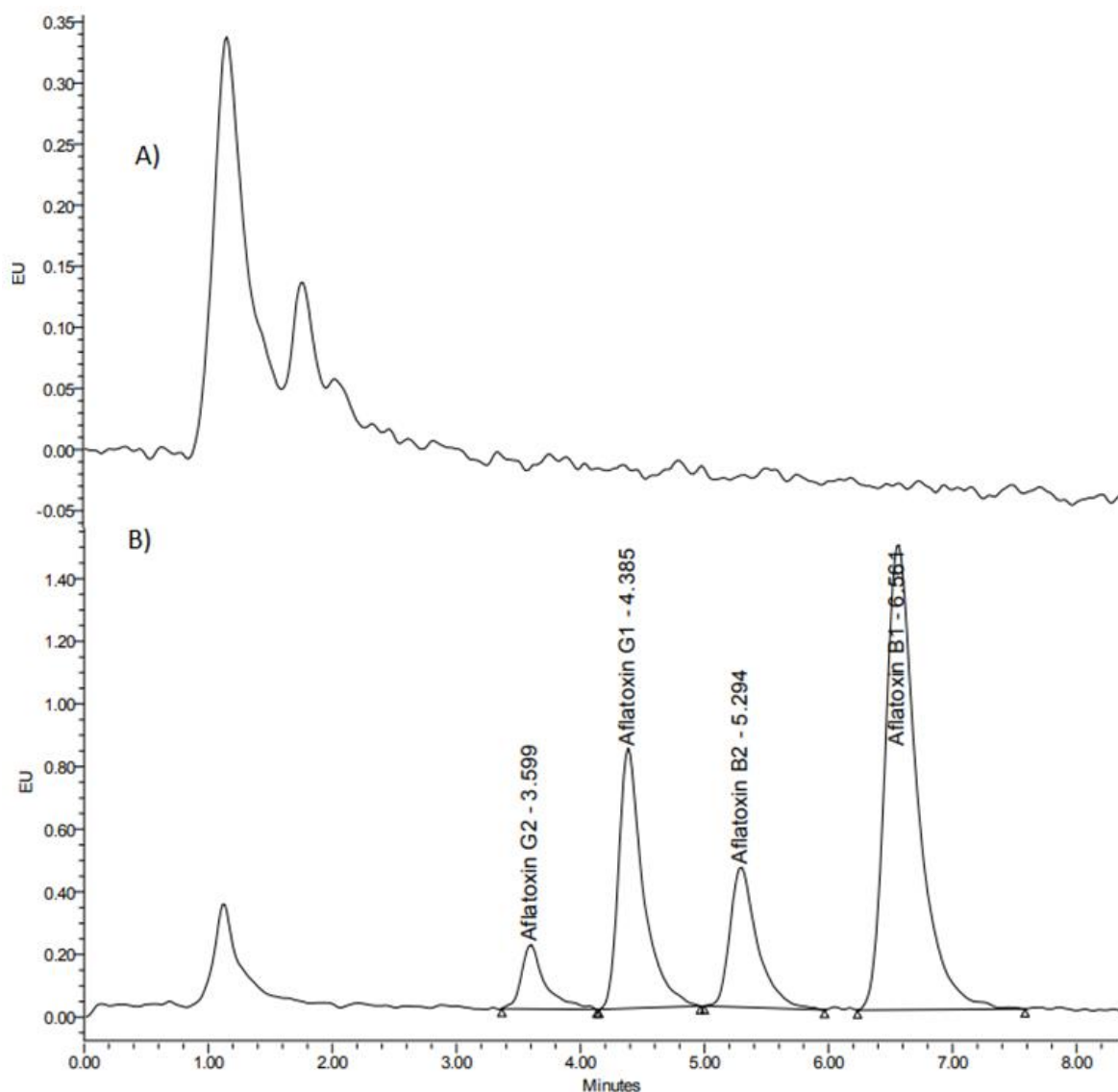
شکل ۲- کروماتوگرام (A): کروماتوگرام نمونه واقعی جمع‌آوری شده از سطح شهر و (B): کروماتوگرام نمونه آلوده شده جای در سطح ۵ ng/g
