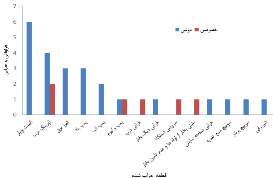
نمودار ۶- فراوانی خرابی قطعات دستگاه بی خطر ساز پسماند در بیمارستان های دولتی و خصوصی استان گلستان در سال ۱۴۰۲
