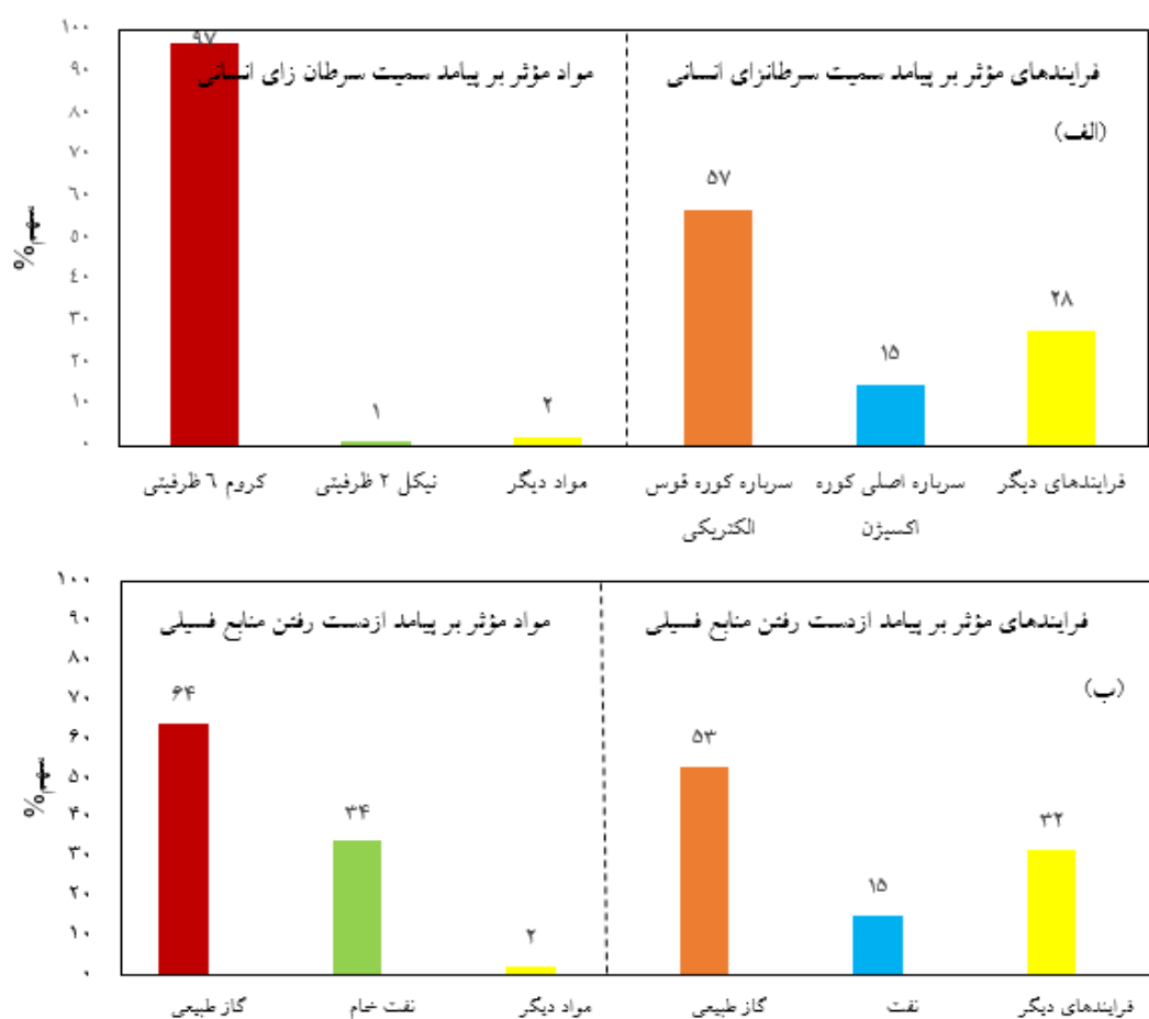
شکل ۲- مواد و فرایندهای مؤثر بر پیامدهای سمیت سرطان‌زای انسانی (الف)، پرغذایی اکوسیستم آب شیرین (ب) و از دست رفتن منابع فیلی (ج) در نیروگاه مورد مطالعه
