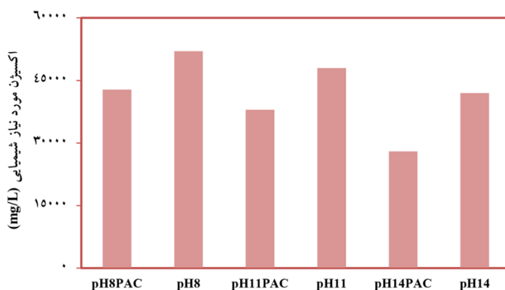
نمودار ۱- COD مربوط به پساب خروجی از مرحله انعقاد و لخته سازی در شرایط مختلف
