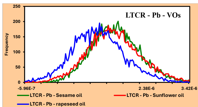
شکل ۳- کران بالا و کران پایین عدم قطعیت (صدک‌های ۹۵th و ۵th) LTCR مربوط به غلظت کل HMs در VO
