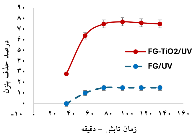
شکل ۷- اثر زمان تابش فرابنفش بر میزان حذف بنزن (۳۹ ppm) با استفاده از فوم شیشه پوشش داده شده با \text{TiO}_2 در
