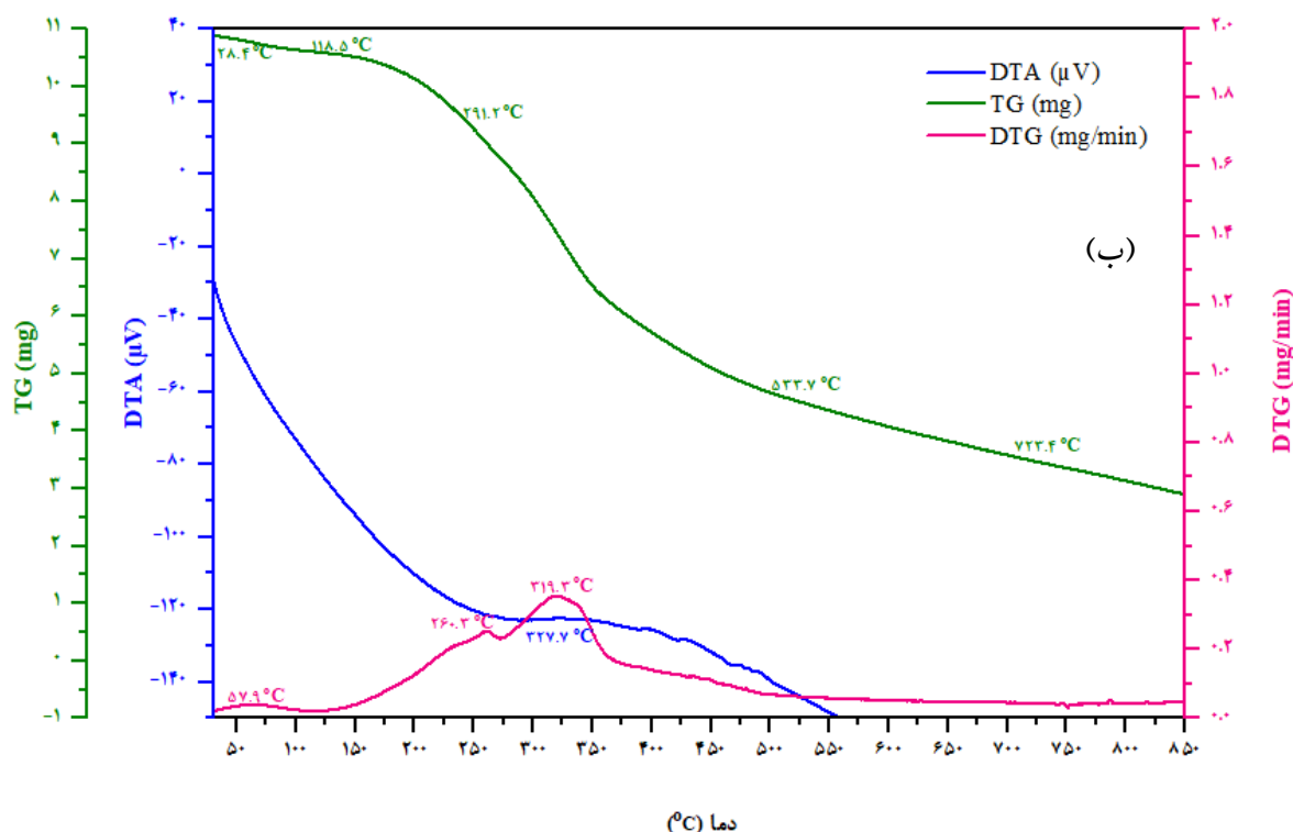
ادامه نمودار ۳- منحنی آنالیز توزین حرارتی الف) SCG و ب) هیدروچار حاصله در شرایط بهینه (۲۳۵ °C، ۱۸۰ min و نسبت L:S:۱:۸)
