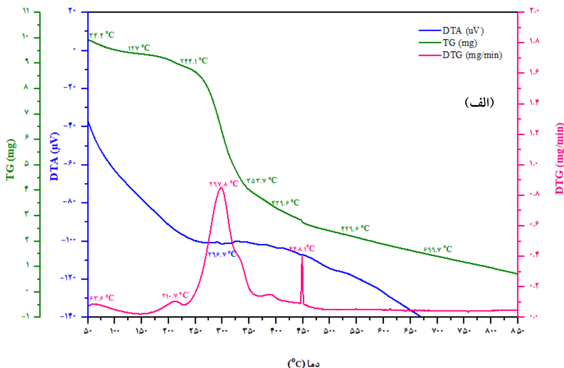
نمودار ۳- منحنی آنالیز توزین حرارتی الف) SCG و ب) هیدروچار حاصله در شرایط بهینه (۲۳۵ °C، ۱۸۰ min و نسبت L:S (۸:۱))
