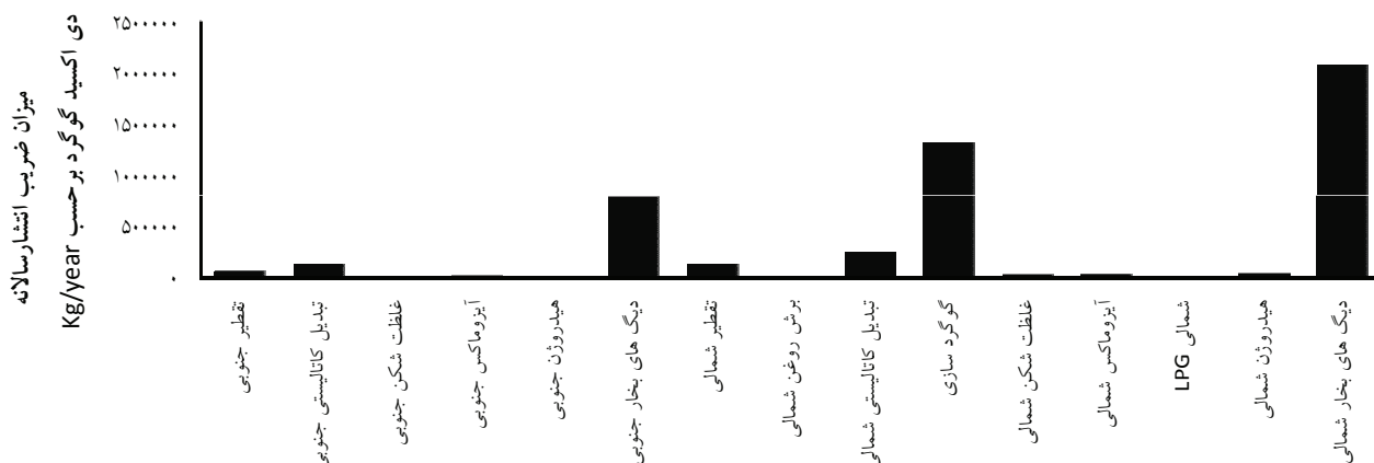
شکل ۳: میزان انتشار سالانه دی اکسید گوگرد تولیدی در واحدهای مختلف پالایشگاه نفت تهران بر حسب (kg/year) واحدهای مختلف پالایشگاه نفت تهران
