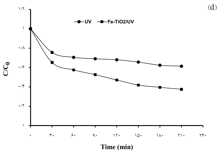
شکل ۹: بررسی مقایسه ای تجزیه فنل با استفاده از UV به تنهایی و فرایند \text{Fe}^{+2}\text{-TiO}_2/\text{UV} در (a) \text{pH}=3 غلظت ۵ میلی گرم در لیتر فنل، (b) غلظت ۱۰ میلی گرم در لیتر فنل، (c) غلظت ۵۰ میلی گرم در لیتر فنل، (d) غلظت ۱۰۰ میلی گرم در لیتر فنل
