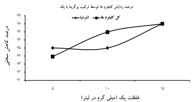
شکل ۶: راندمان زدایش کلیفرم ها
