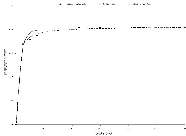
شکل ۶: برازش مدل‌های سینتیک جذب سرب توسط جاذب جاذب میلی‌متری خاکستر برگ سدر (غلظت محلول فلزی ۱۰ میلی‌گرم بر لیتر، مقدار جاذب ۱۰ گرم بر لیتر، pH=۵)
