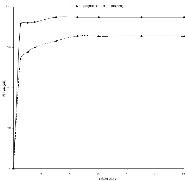
شکل ۴: تاثیر زمان تماس بر جذب سرب (مقدار جاذب، ۱۰ گرم بر لیتر، غلظت اولیه محلول ۱۰ میلی گرم بر لیتر و pH=5 )
