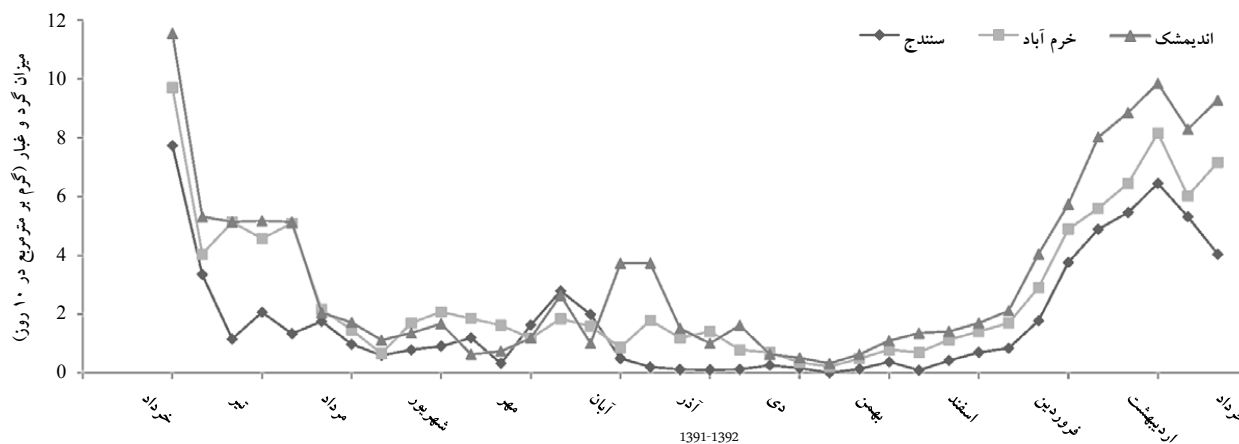
شکل ۲: روند تغییرات میزان ذرات گرد و غبار باریده بر سه شهر سنندج، خرم آباد و اندیمشک در طول دوره نمونه‌برداری (gr/m 2 .10 days)
