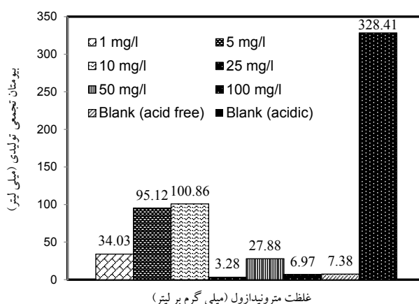
شکل ۷: میزان تولید تجمعی متان‌سازی ویژه جرم زیستی بی‌هوازی با تاثیر داروی مترونیدازول قبل از پیش تصفیه با فرایند UV_{254}/H_2O_2 در غلظت‌های ۱، ۵، ۱۰، ۲۵، ۵۰، ۸۰ mg/L
