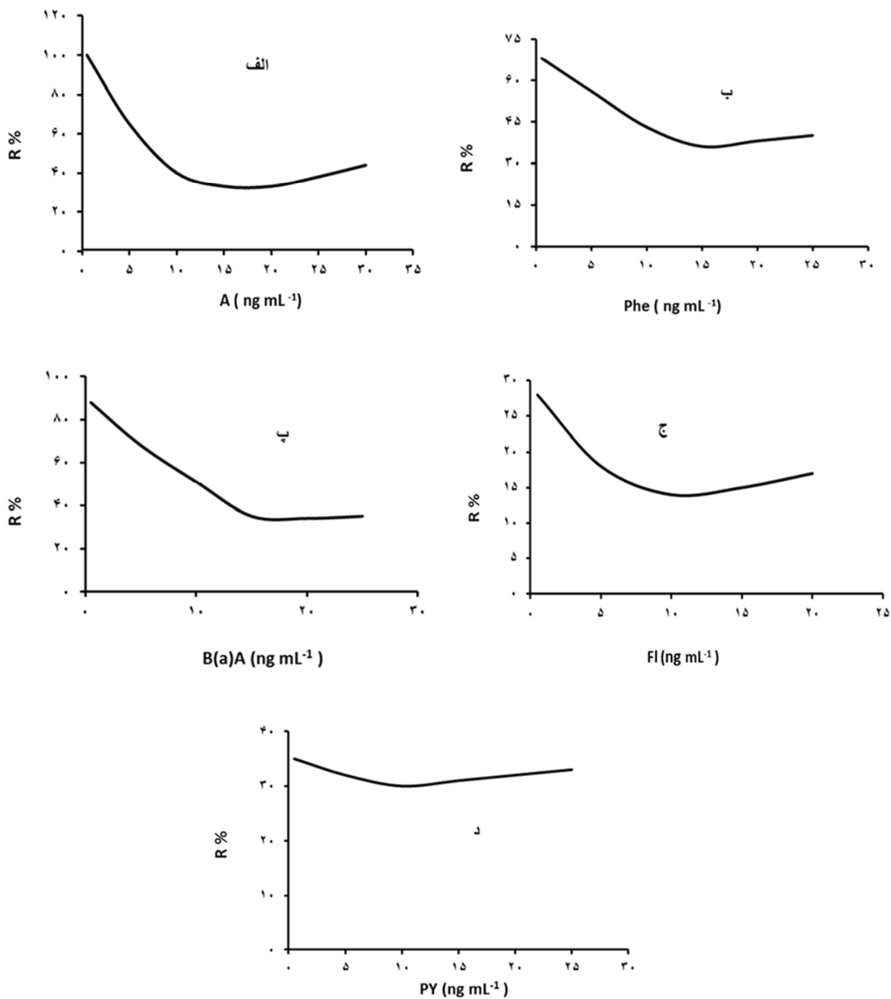
شکل ۴: متحنی کالبراسیون (الف) آنتراسن (ب) فناترون (پ) بنز (a) آنتراسن (ج) فلورن (د) پیرن در شرایط بهینه بر اساس %R نسبت به غلظت PAHs.
