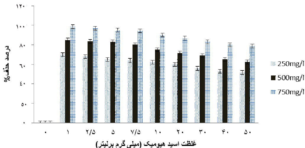
شکل ۴: تاثیر غلظت‌های مختلف نانوذرات اکسید آهن پوشش داده با سیلیس بر غلظت‌های مختلف اسید هیومیک در pH ۱۰/۵ و زمان 90 min
